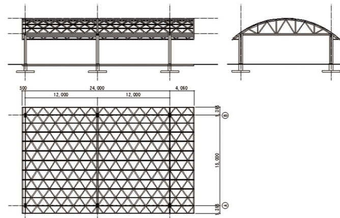
吊り込み：シェル屋根
