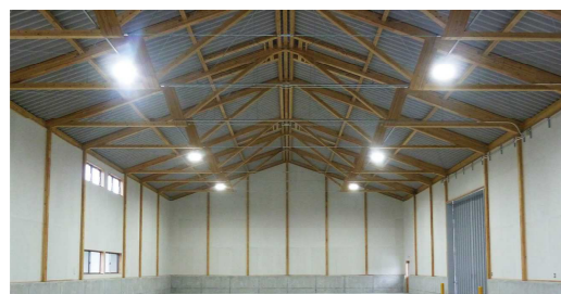
構造: 木造平屋 スパン15m 施工面積: 450 m 2
