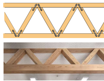
トラス梁
