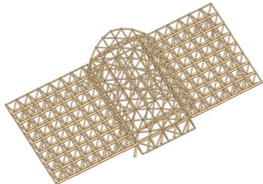
吊り込み：シェル屋根
