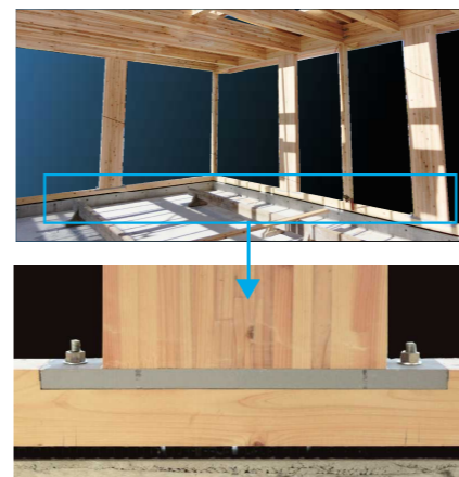
木造2階建て店舗 (EH450使用)
