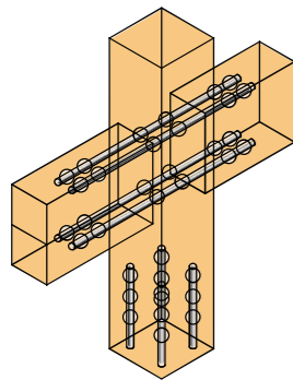
ラーメン構造
