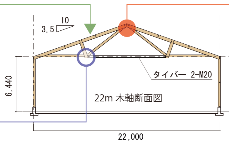
工場組立・現場搬入トラス トラスは、搬入サイズまでは組み立てた状態で納品します。
