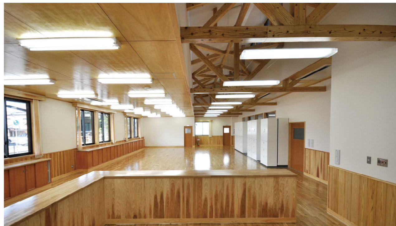
拡張樹脂アンカー工法使用
