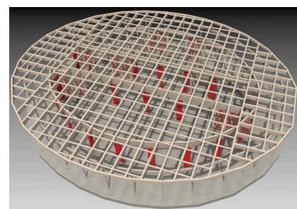
木軸鳥観図
