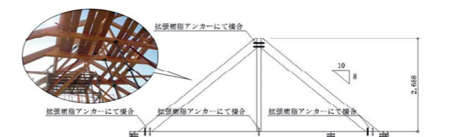
拡張樹脂アンカー工法使用
