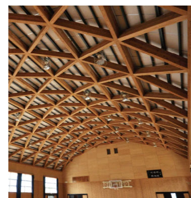
木造軸組
