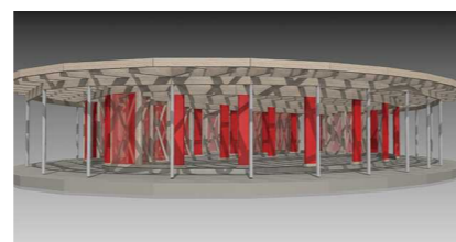
外観軸組(パース)
