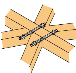
ラチスシェル
